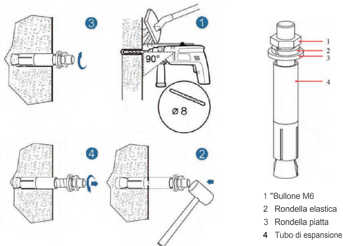
Figura 6-4 Installazione del bullone di espansione (unità: mm)
