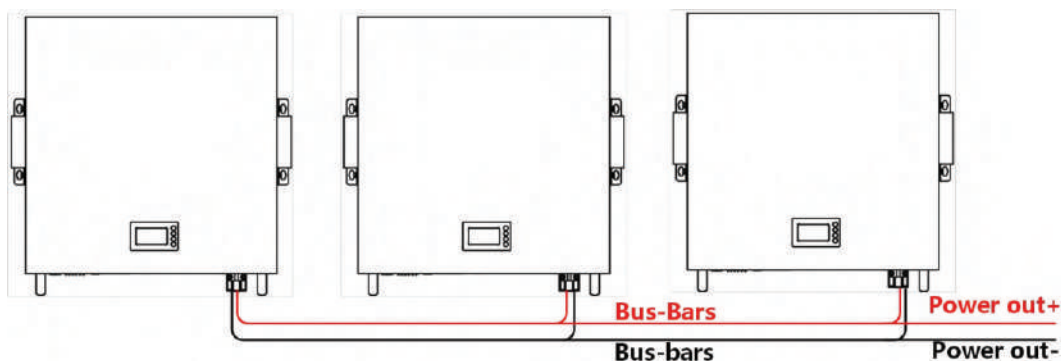
Figura 6-6 Collegamento del cavo di alimentazione del gruppo batteria alle sbarre colletttrici
